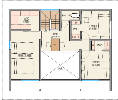
2階平面図
