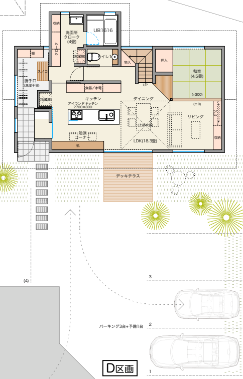
1階平面配置図
